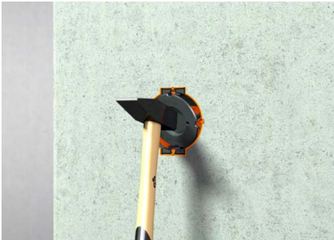
Deckel durch einen einfachen Hammerschlag öffnen.
