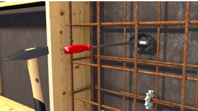
Mithilfe integrierter Wasserwaage ausrichten und aufnageln.
