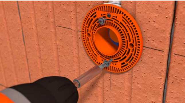
Schrauben finden im Geräteträger eine passende Öffnung und Halt.
