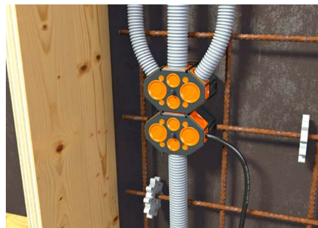
Werkzeuglose Kombi-Einführung weiterer Kabel und Rohre M15 – M32. Einführung von starren Rohren möglich.
