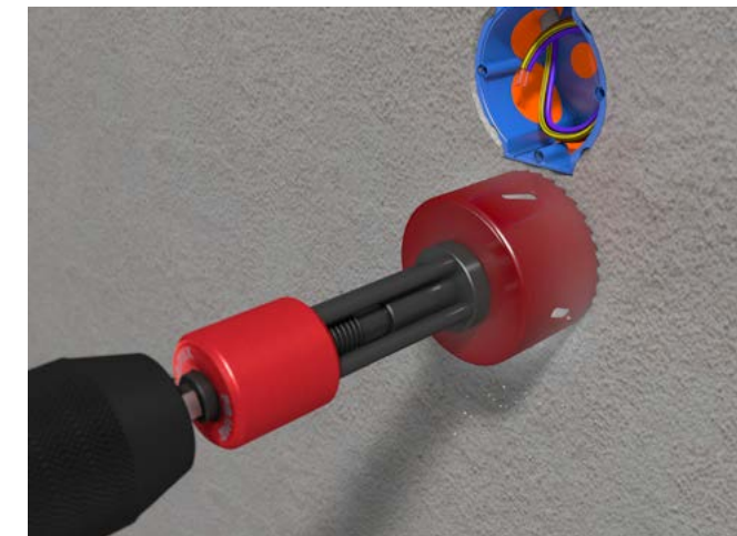
... oder mit einer Bohrkrona aufgebohrt werden.
