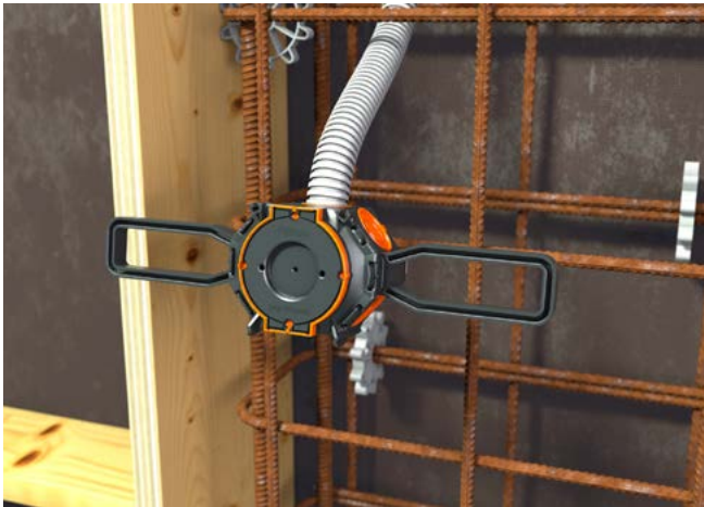
Flügel auf die Membrandose stecken.
