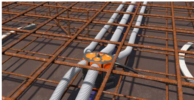
Zweite Stahlarmierung legen.
