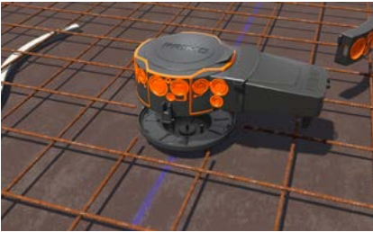
Kurzer Trafotunnel kann durch Universaltrafotunnel für zusätzlichen Installationsraum ersetzt werden.
