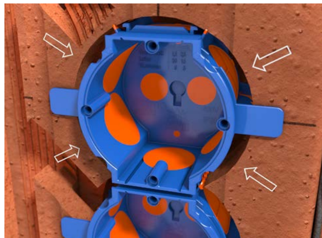
Passgenau durch Membranrastzähne.
