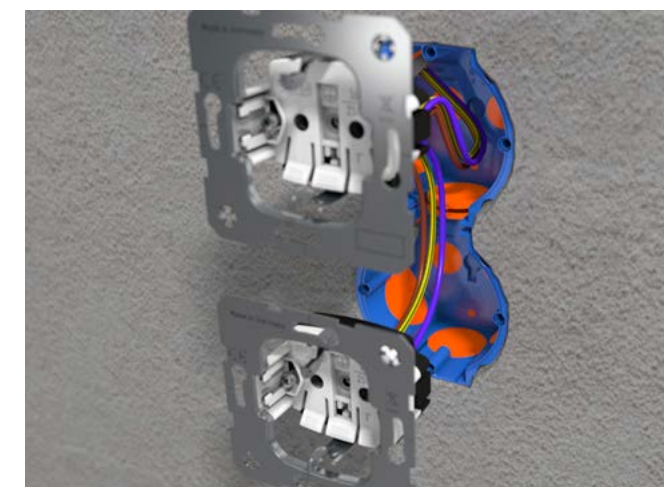
Einfache und zeitsparende Durchgangsverdrahtung sowie Installation von vorverdrahteten Einbaugeräten durch ausbrechen des SCS-Steg möglich.
