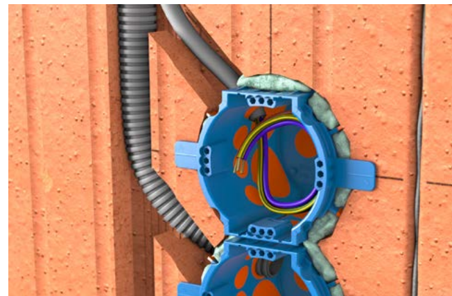
Membrane mit Leitung durchstoßen und einführen.
