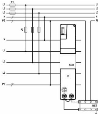
TNS-Netz
