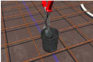
Universaldose mit Nägeln auf die Schalung fixieren. Loch mit Stanzzange ausstanzen.
