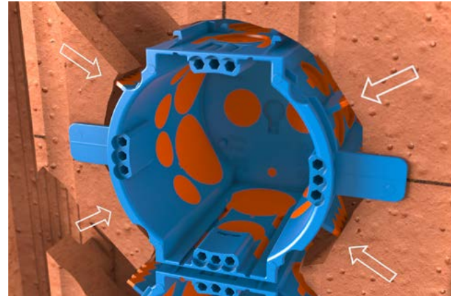
Passgenau durch Membranrastzähne.
