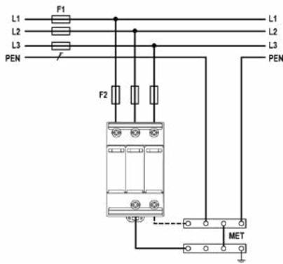
TNC-Netz
