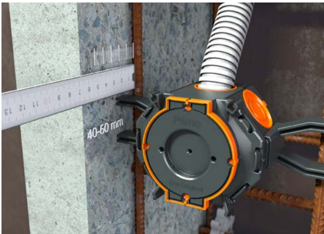
... oder um 180° gedreht für 40 – 60 mm Betonüberdeckung.
