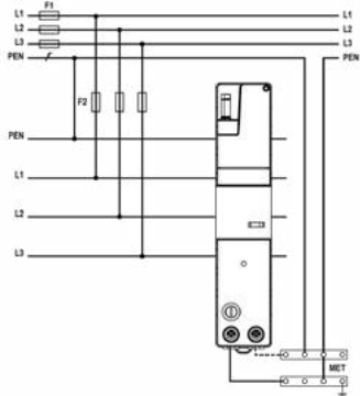
TNC-Netz
