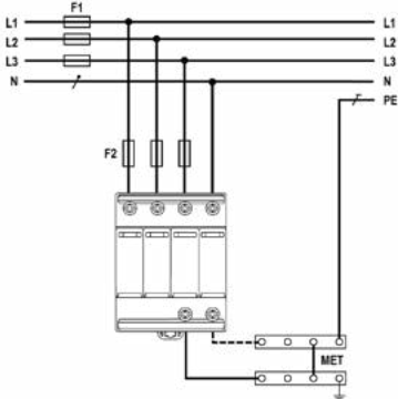
TT-Netz
