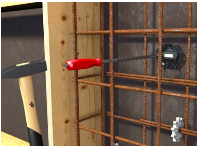
Wurde die zweite Bewehrung bereits angebracht, kann der Deckel mit dem Nagler (P752) positioniert und aufgenagelt werden.
