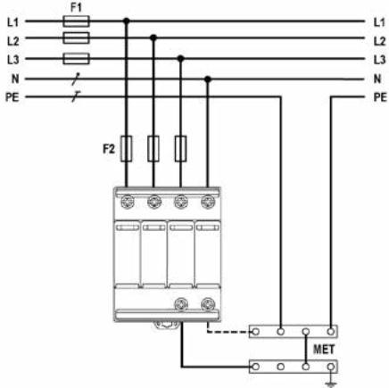
TNS-Netz
