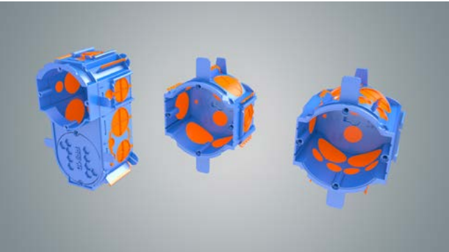
Alle Therm Dosen lassen sich miteinander kombinieren.
